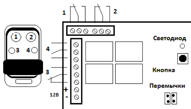
Рис.2 Схема включения и органы управления
